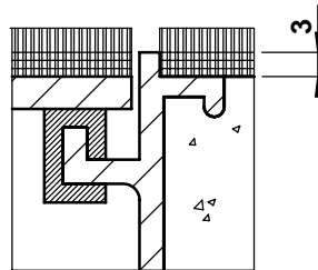
détail a
