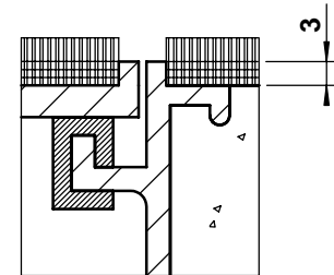
détail a 2
