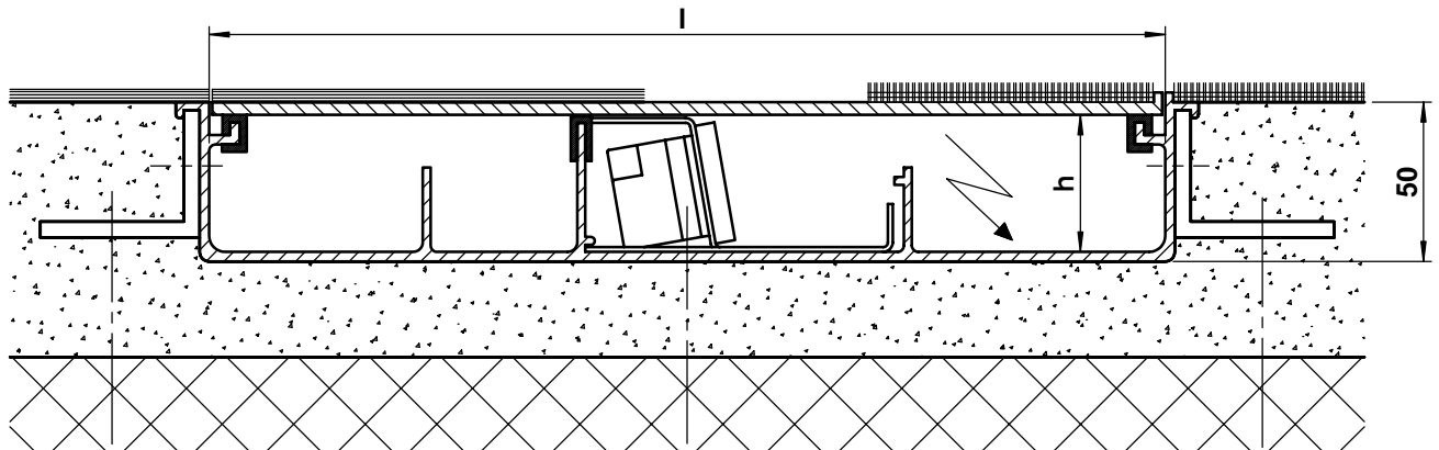
détail s
