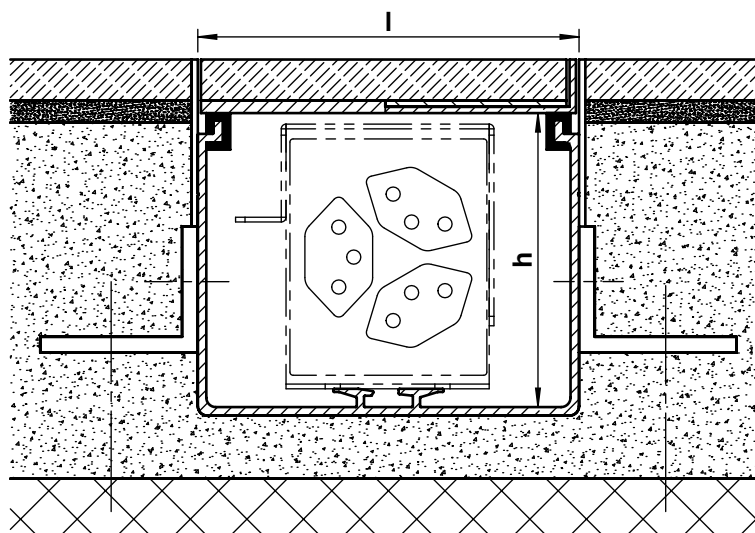
détail a
