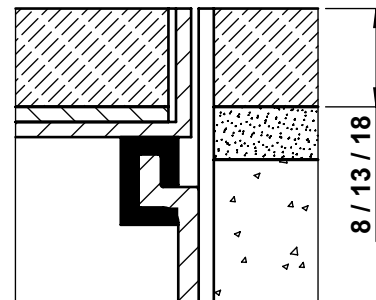
détail a 2
