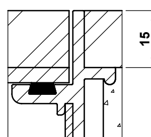
détail a
