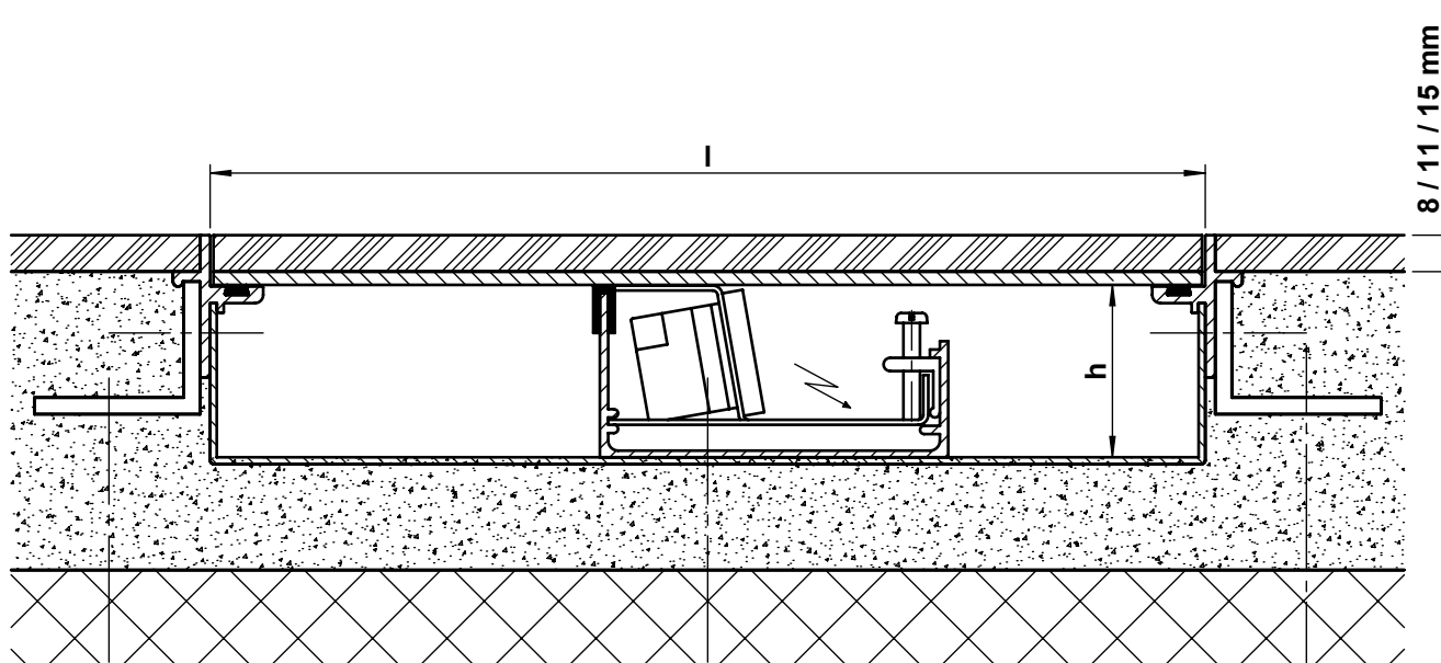
détail a
