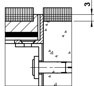
détail a 2
