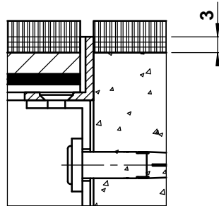
détail a
