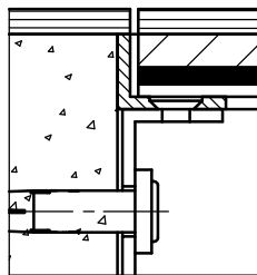
détail s
