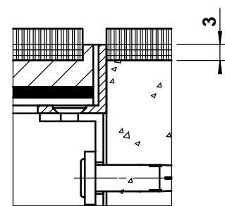
détail a 2
