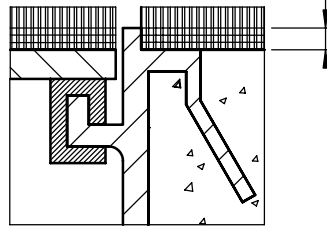
détail a
