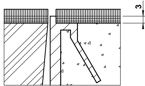
détail a
