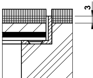
détail a
