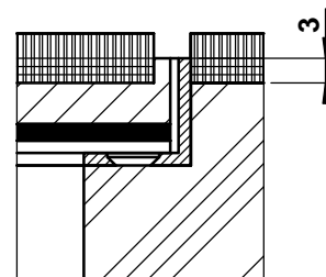
détail a 2
