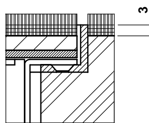
détail a
