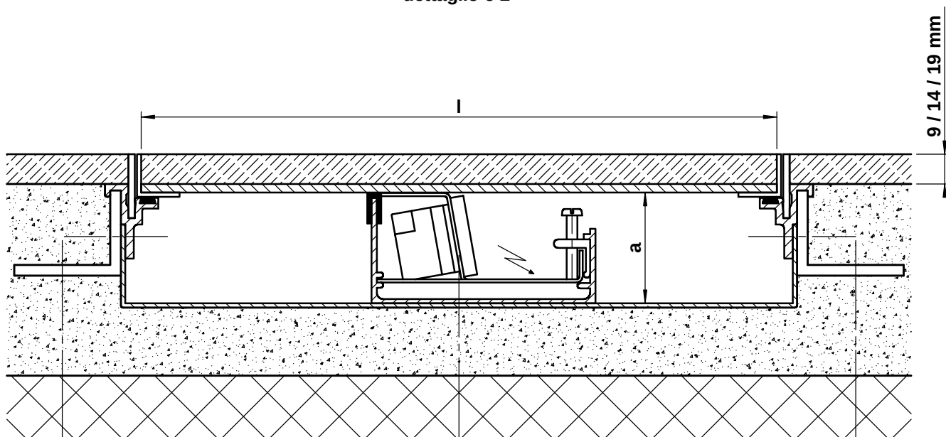
dettaglio c 2
