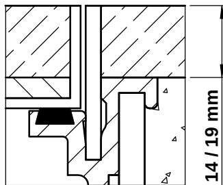
dettaglio c 2
