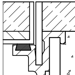
dettaglio c 2
