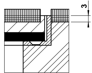
dettaglio c 2
